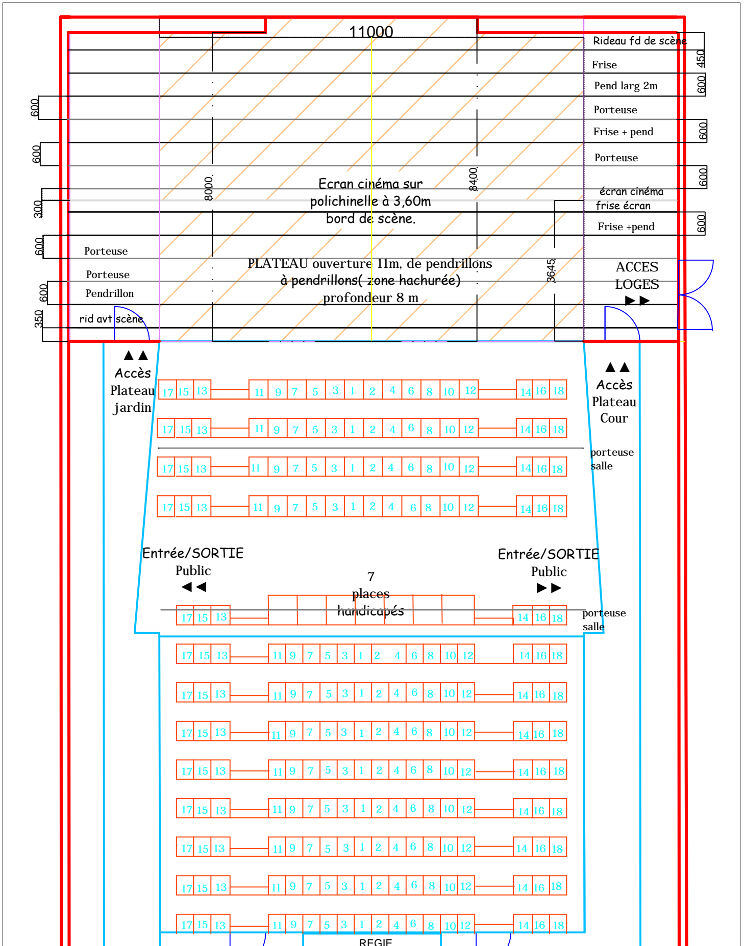
Plan salle de spectacle du LISSIACO échelle 1/100
